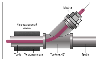
Монтаж кабеля в трубу через тройник 45°
