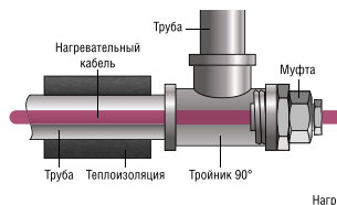
Схема 1. Монтаж муфты в тройник 45°
