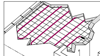
Размещение кабеля на подъездных путях
